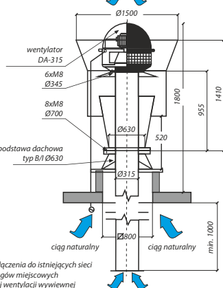
Wywietrzak zintegrowany WZ-630/DA-315
